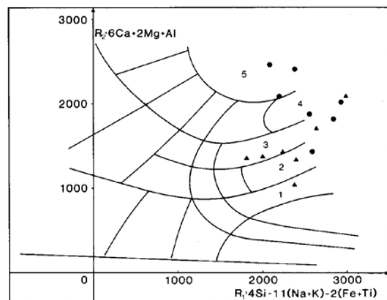
Fig. 8: De la Roche R_1R_2 -diagram van die hornblendiet (●) en die mafiese fase van die Violdsdriftsuite (▲) — (1) tonaliet, (2) dioriet, (3) gabbro-dioriet, (4) gabbro-noriet en (5) ultramafiese gesteentes.
